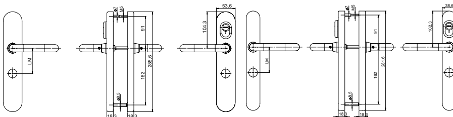
Kaba c-lever Standard-Ausführung. Breites und schmales Schild, Schweizer Profil. Typ 2622 und 2621.
